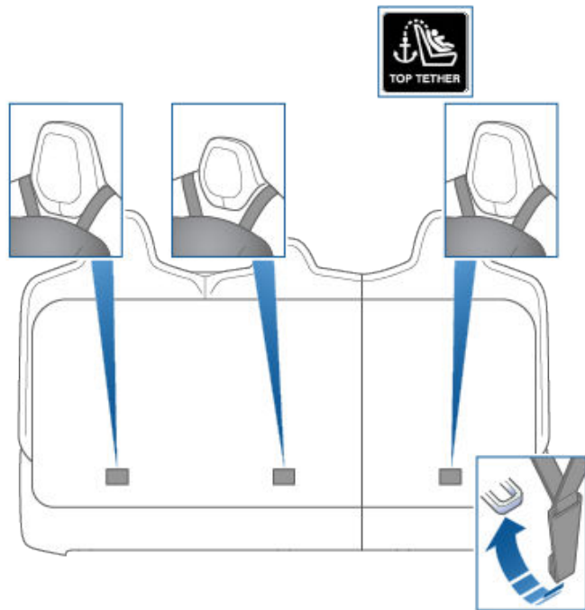
Dva popruhy – sedadla ve třetí řadě
